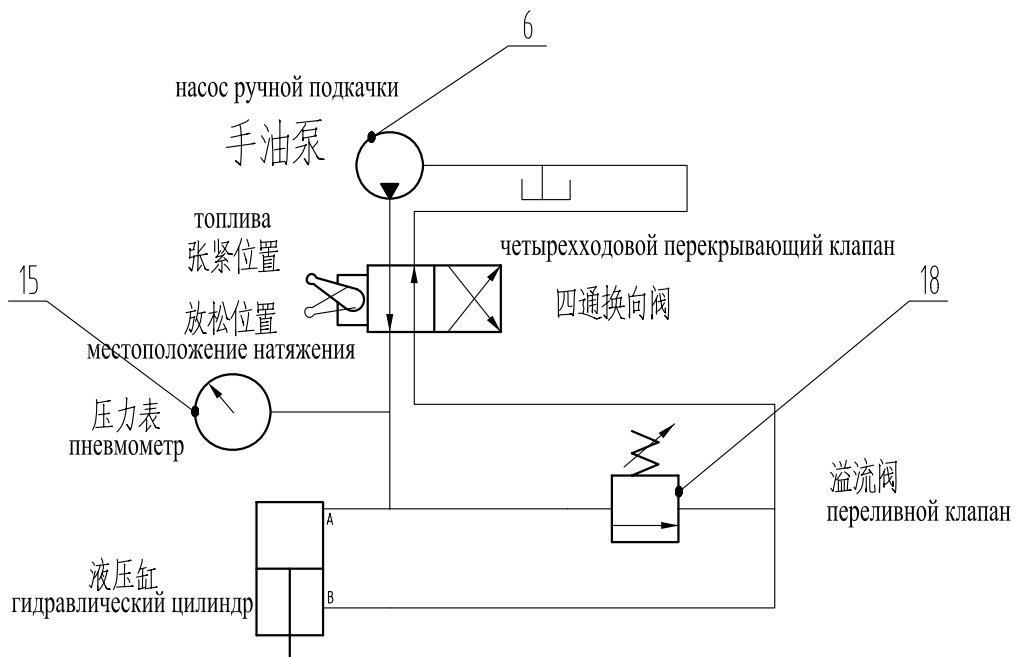
皮带张紧液压原理示意图 Схема гидравлического принципа натяжения ремня
